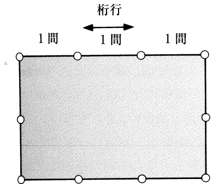
図3 「桁行3間・梁行2間」の平面
